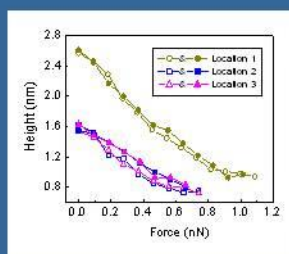
单个DNA分子的压力弹性表征
