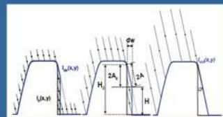
原子力显微镜成像标准化
